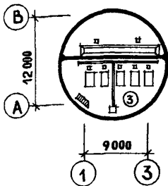
ПЛАН НА ОТМ. -9,240; -9,250
