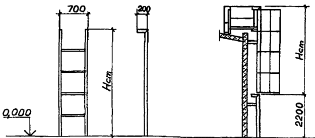
КОМПОНОВОЧНЫЕ СХЕМЫ СТРЕМЯНОК И ОГРАЖДЕНИЙ СТРЕМЯНОК
