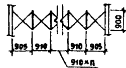
Кабины душевых закрытые однорядные
