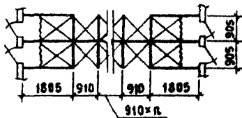
Кабины душевых открытые и закрытые двухрядные
