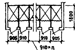
Кабины душевых закрытые однорядные
