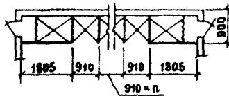
Кабины душевых открытые и закрытые однорядные
