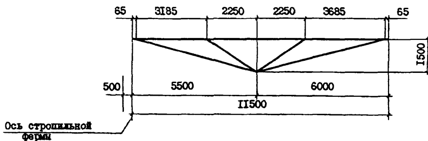
Схема прогонов типа ПК-, ПКС-
