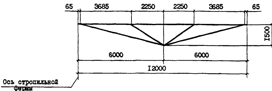
Схема прогонов типа ПК-, ПКС-
