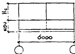
I-I фонарные панели при шаге ферм 6 м при шаге ферм 12 м
