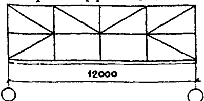
2-2 ветрозащитные панели при шаге ферм 6 и 12 м
