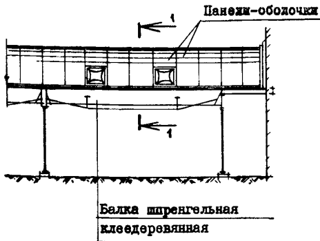
Надземная галерея
