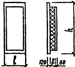
НОМЕНКЛАТУРА СТЕНОВЫХ ПАНЕЛЕЙ
