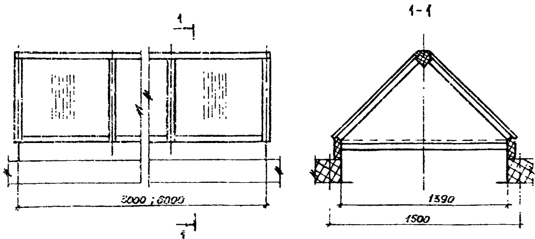
Пример компоновки фонарей на кровле
