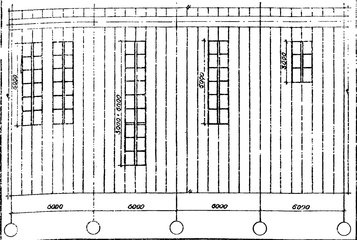
Пример компоновки фонарей на кровле
