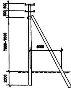
Угловые анкерные
