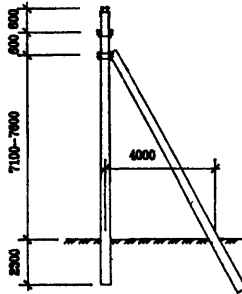
Концевые (анкерные)
