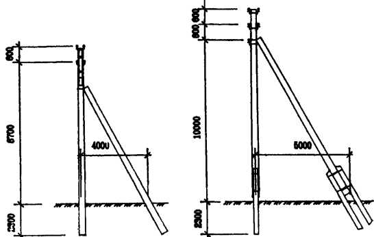
Концевые
