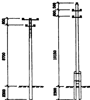
Промежуточные
