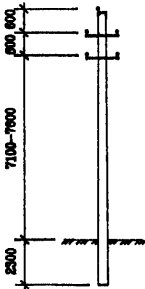
Промежуточные
