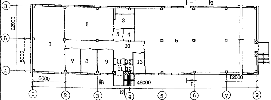
ЭКСПЛИКАЦИЯ ПОМЕЩЕНИЙ
