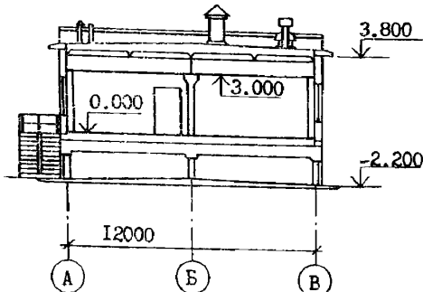
РАЗРЕЗ I-I
