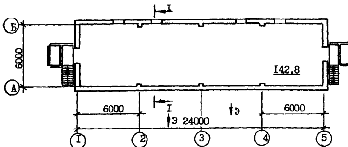
ПЛАН НА ОТМЕТКЕ 0.000
