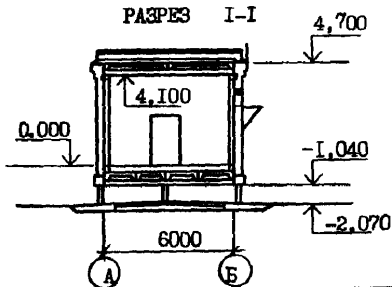
РАЗРЕЗ I-I
