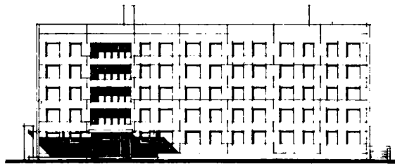
ФАСАД I-10
