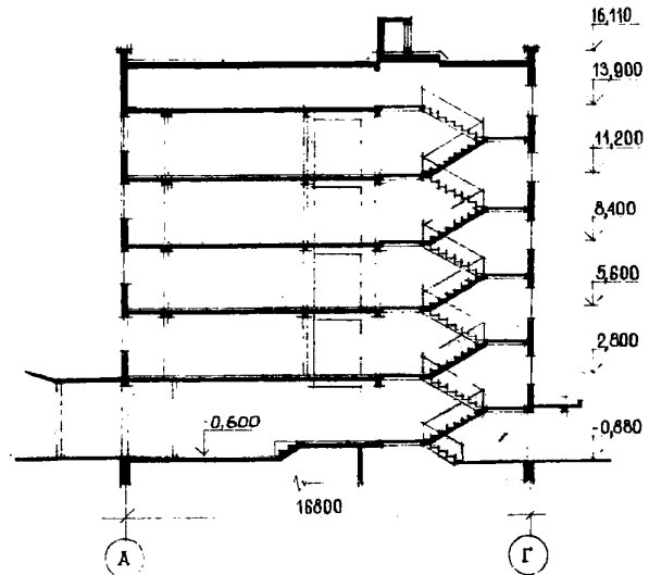
РАЗРЕЗ I-I
