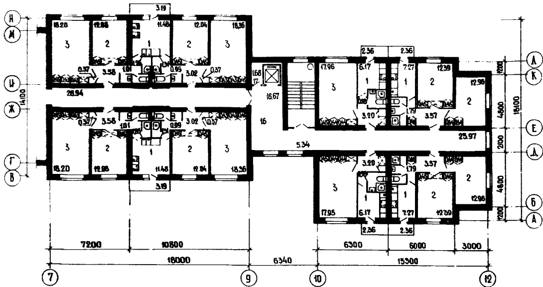
ЭКСПЛИКАЦИЯ ПОМЕЩЕНИЙ
