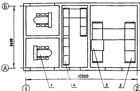
ТЕХНОЛОГИЧЕСКОГО ОБОРУДОВАНИЯ
