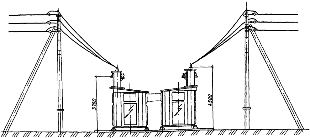
ПРИСОЕДИНЕНИЕ ВЛ 10 и 0,4 кВ К ПОДСТАНЦИИ С ВОЗДУШНЫМИ ВВОДАМИ
