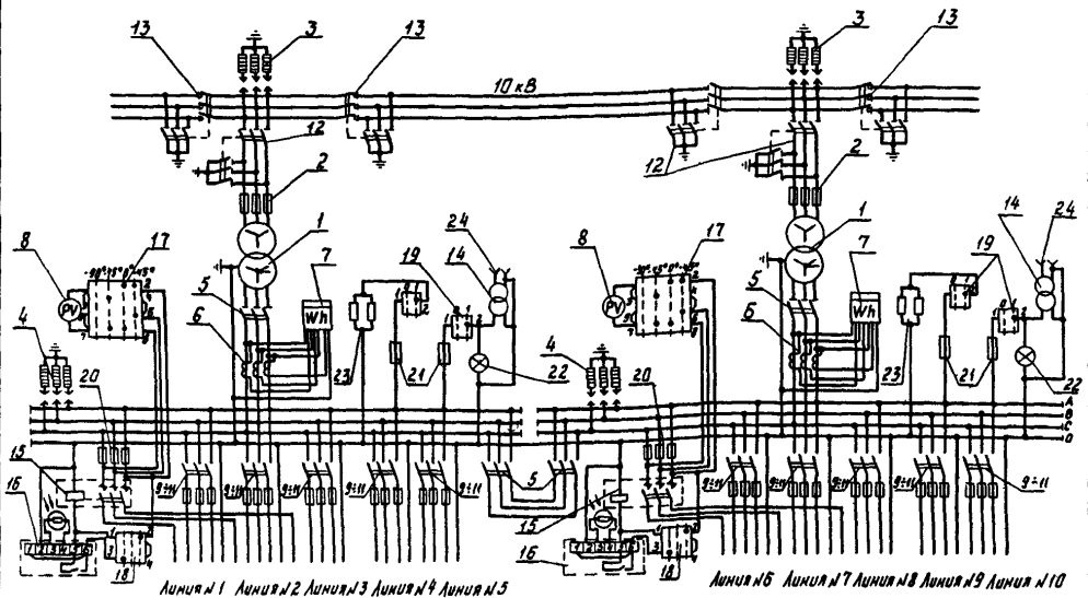
СХЕМА ЭЛЕКТРИЧЕСКИХ СОЕДИНЕНИЙ ПОДСТАНЦИИ
