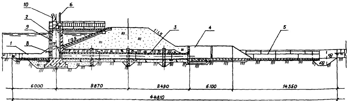
РАЗРЕЗ I-I
