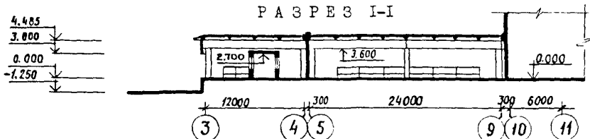
РАЗРЕЗ I-I
