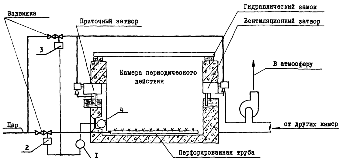
СХЕМА
