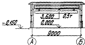
РАЗРЕЗ I-I
