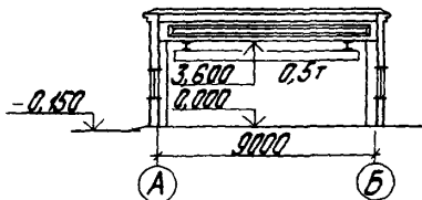
РАЗРЕЗ 2-2
