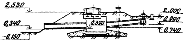
РАЗРЕЗ I-I
