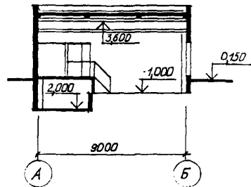
РАЗРЕЗ I-I
