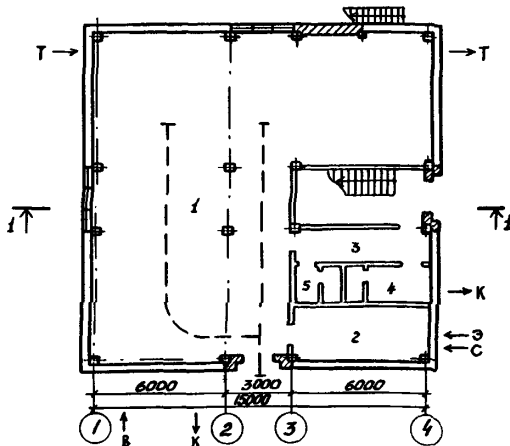
ЭКСПЛИКАЦИЯ ПОМЕЩЕНИЙ
