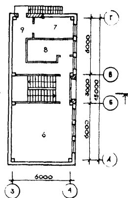
ПЛАН НА ОТМ. 3.300
