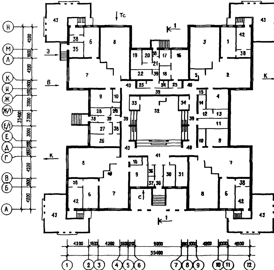
ПЛАН ЭТАЖА
