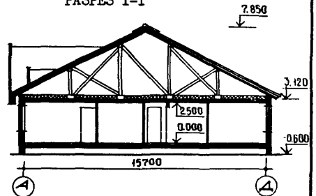
РАЗРЕЗ I-I
