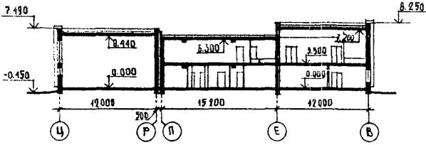
РАЗРЕЗ 3-3
