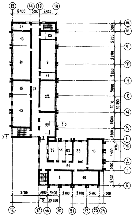
ПЛАН 3 ЭТАЖА
