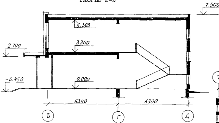
РАЗРЕЗ 2-2
