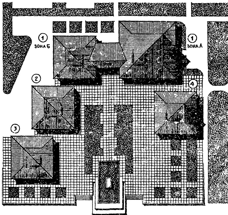
СХЕМА ГЕНПЛАНА
