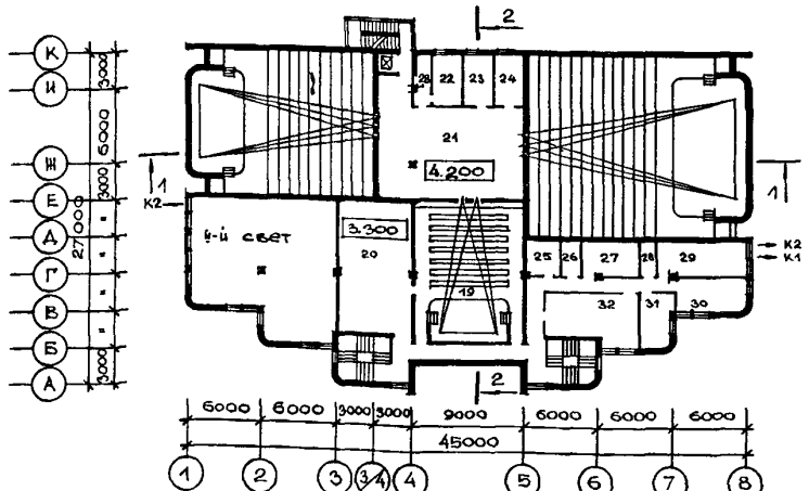
ПЛАН 2 ЭТАЖА
