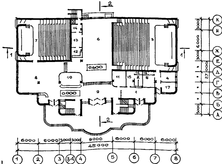
ПЛАН 2 ЭТАЖА
