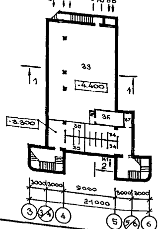
ПЛАН ПОДВАЛА
