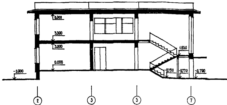
РАЗРЕЗ I-I
