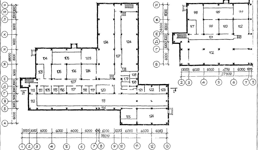
ПЛАН НА ОТМ. -2.800 /ВАРИАНТ/
