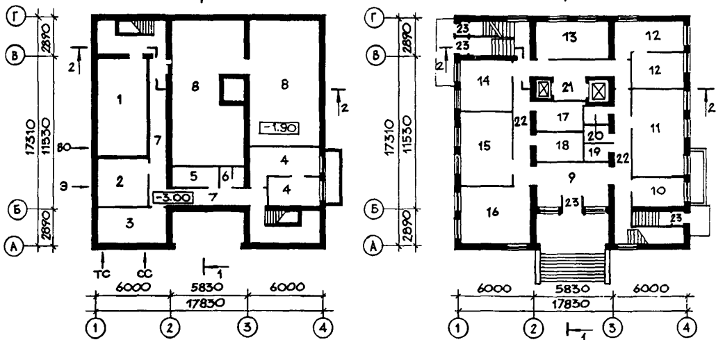
ЭКСПЛИКАЦИЯ ПОМЕЩЕНИЙ
