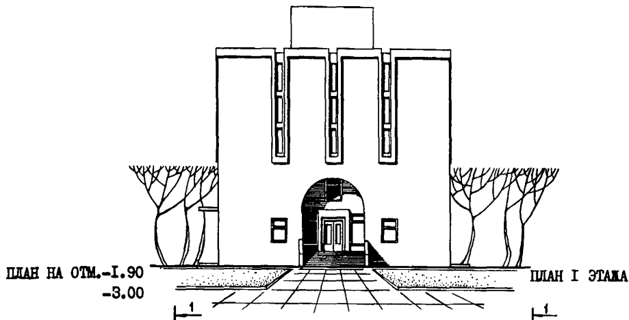
ФАСАД I-4
