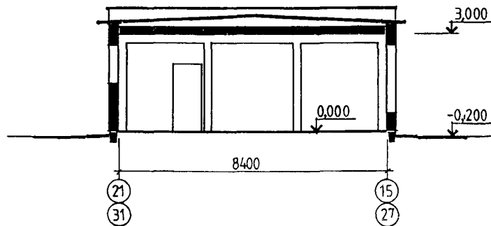
РАЗРЕЗ I-I
