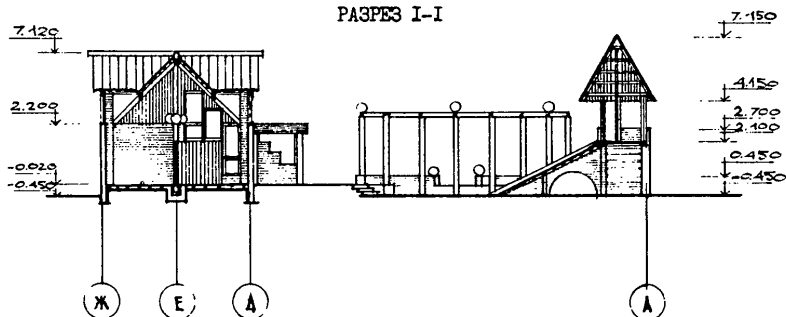
РАЗРЕЗ I-I
