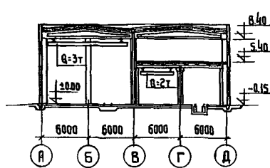
РАЗРЕЗ I-I
