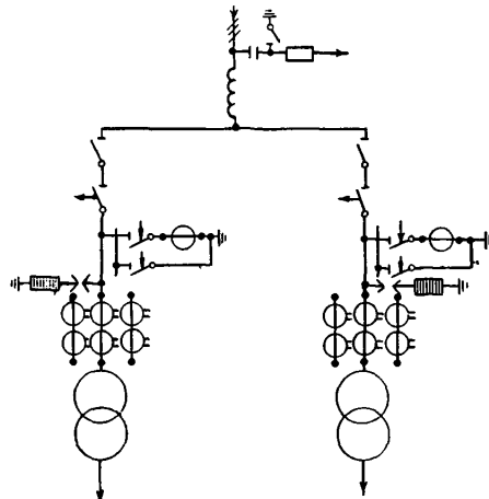
СХЕМА ЭЛЕКТРИЧЕСКИХ СОЕДИНЕНИЙ ПОДСТАНЦИИ СО СТОРОНЫ 10 КВ
