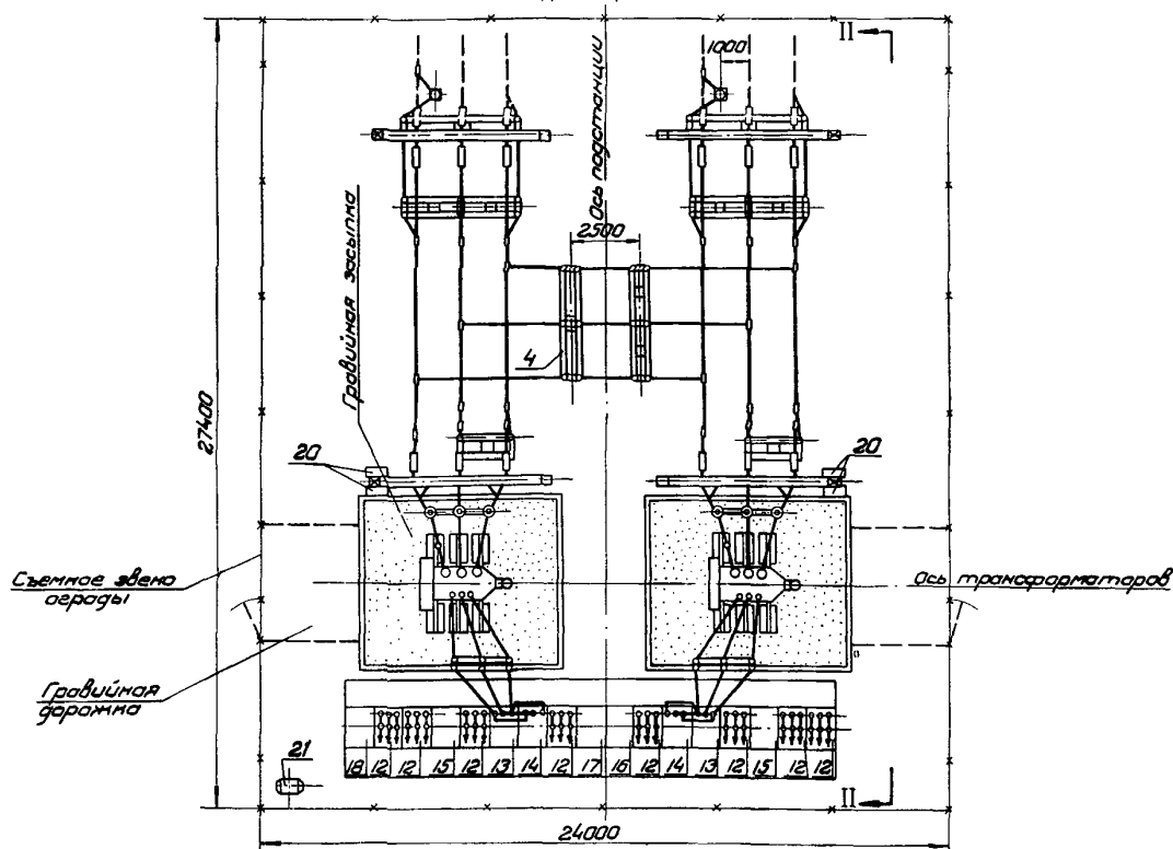
ПЛАН ПОДСТАНЦИИ
