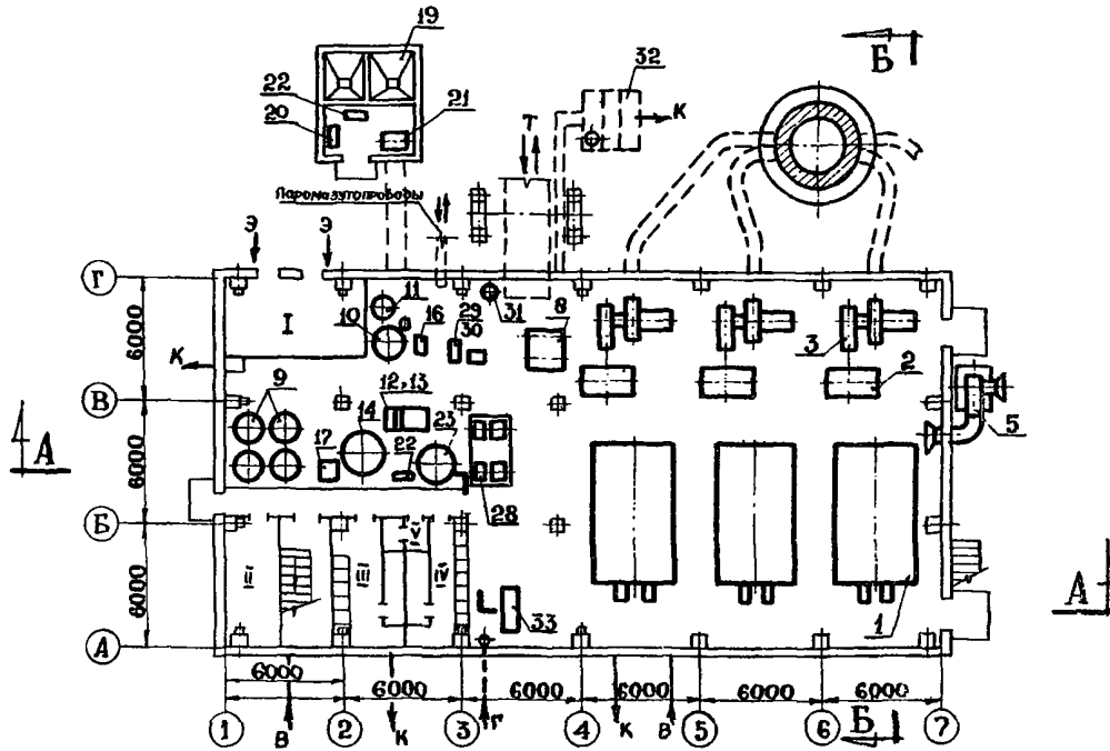
ПЛАН НА ОТМ. \pm 0,00
