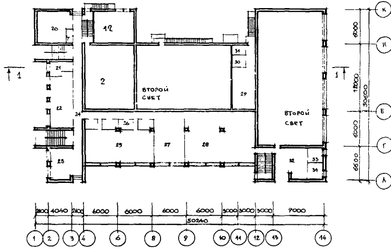
ПЛАН 2-го ЭТАЖА
