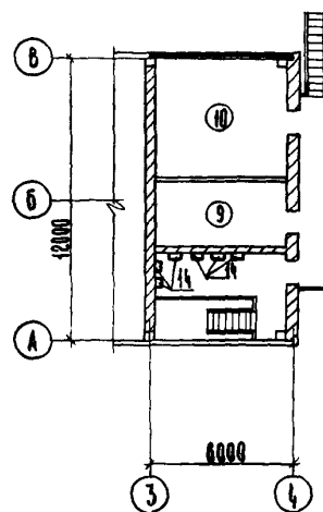
ЭЛЕМЕНТ ПЛАНА НА ОТМ. 3.30
