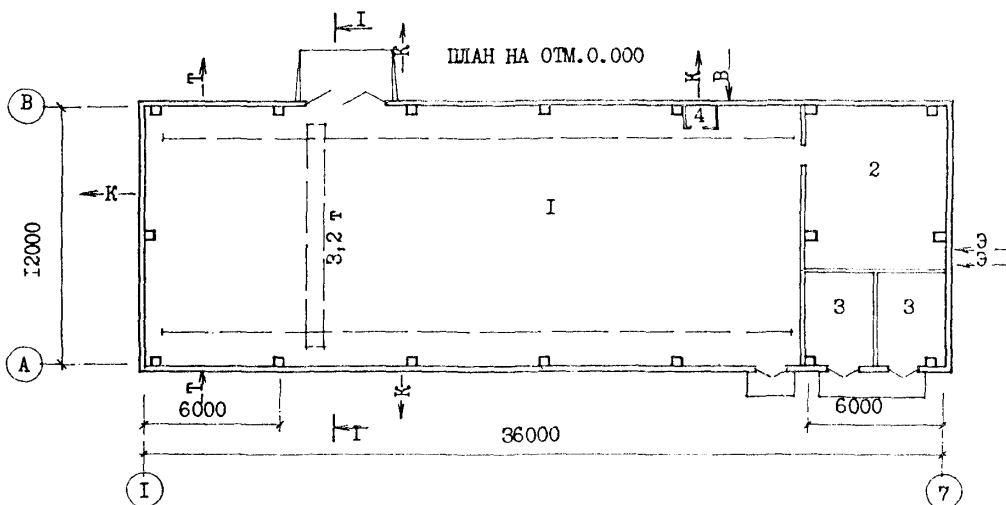
РАЗРЕЗ I-I
