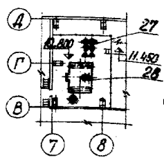
ПЛАН НА ОТМ. 10.800 открытая система
