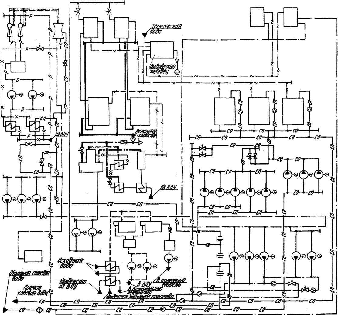
ТЕПЛОВАЯ СХЕМА КОТЕЛЬНОЙ /вариант для открытой системы теплоснабжения/
