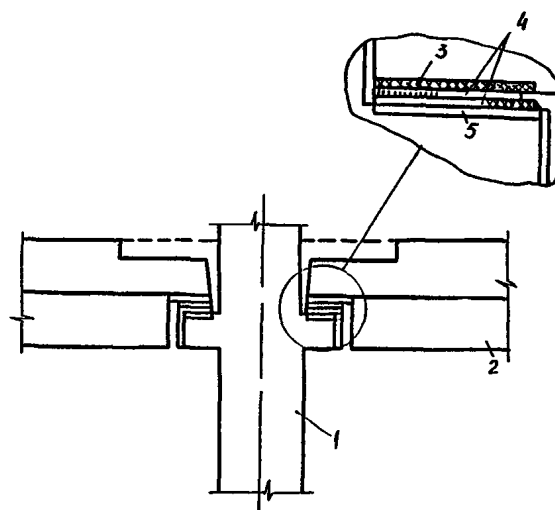
Черт. 2. Конструкция узла сопряжения ригелей с колонной
