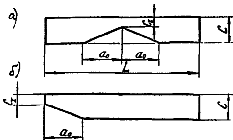
Черт. 5. Схемы изменения жесткости основания в грунтовых условиях I типа по просадочности а — замачивание основания под серединой здания (сооружения); б — то же, под торцом
