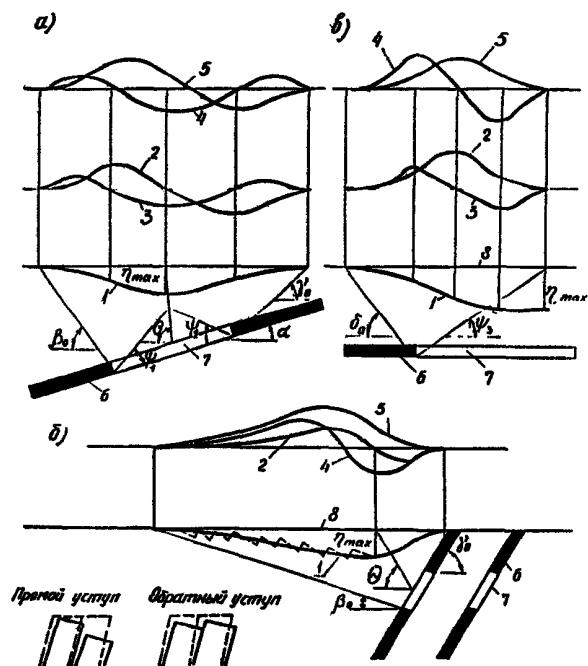
Черт. 1. Виды сдвижений и деформаций земной поверхности а — вертикальный разрез вкрест простирания при наклонном залегании угольных пластов; б — то же, при крутом залегании угольных пластов; в — вертикальный разрез по простиранию пластов; 1 — кривые оседаний; 2 — эпюры наклонов; 3 — эпюры кривизны; 4 — эпюры относительных горизонтальных деформаций; 5 — эпюры горизонтальных сдвижений; 6 — пласт; 7 — очистная выработка; 8 — положение земной поверхности до подработки; \eta_{max} — максимальное оседание земной поверхности; \beta_0 , \gamma_0 , \delta_0 — граничные углы сдвижения; \psi_1 , \psi_2 , \psi_3 — углы полных сдвижений; \theta — угол максимального оседания; \alpha — угол падения пласта
