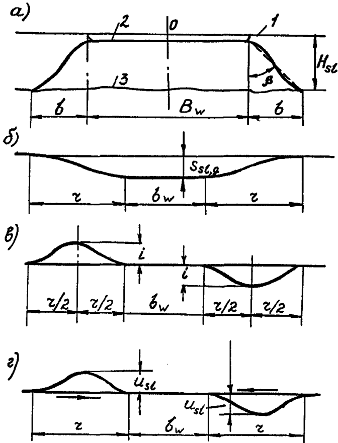
Черт. 2. Характер развития деформаций земной поверхности в пределах просадочной воронки a — поперечный разрез зоны увлажнения; b — кривая просадки поверхности грунта; \epsilon — кривые наклонов поверхности; z — кривые горизонтальных перемещений поверхности грунта; 1 — положение земной поверхности; 2 — площадь замачивания; 3 — нижняя граница растекания воды; b — ширина зоны растекания воды; B_w — ширина замачиваемой площади; \beta — угол растекания воды; H_{sl} — просадочная толщина; r — расчетная длина криволинейного участка просадки грунта от собственного веса; b_w — ширина горизонтального участка просадки; s_{sl,g} — просадка грунта от собственного веса; i — наклон земной поверхности; u_{sl} — горизонтальные перемещения земной поверхности.
