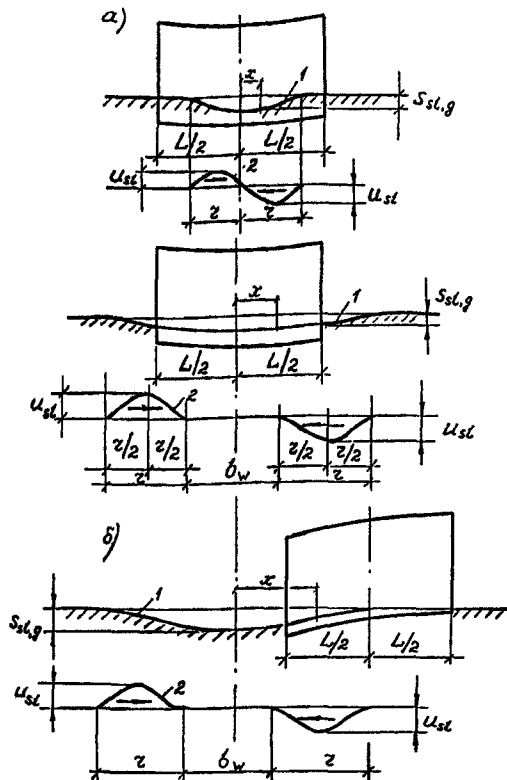
Черт. 4. Схемы вертикальных и горизонтальных перемещений земной поверхности при просадке грунтов от собственного веса
