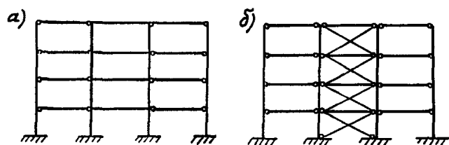
Черт. 1. Схемы рам каркасов многоэтажных зданий а — комбинированной конструктивной системы; б — связевой системы
