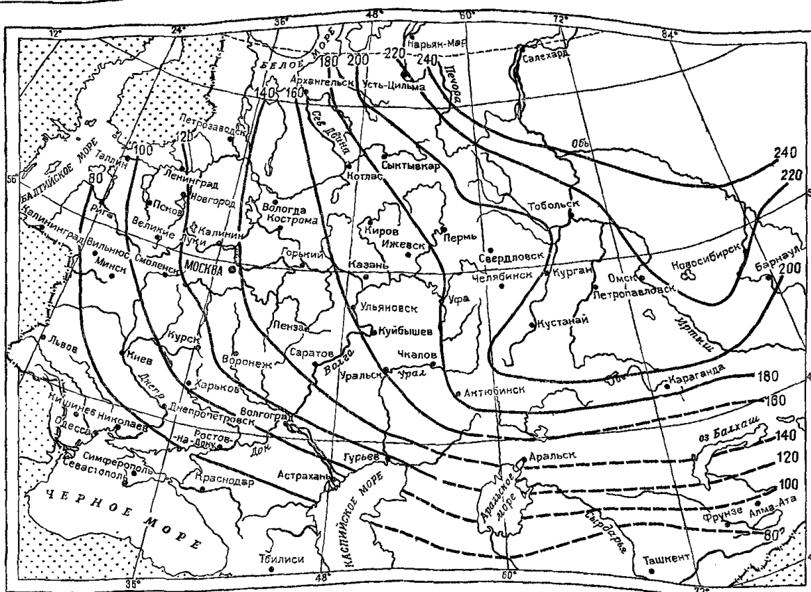
Прил. 1. Рис. 3. Схематическая карта глубины промерзания глинистых и суглинистых грунтов на территории СССР, см
