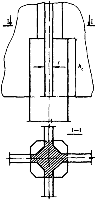
Черт. 9. Заделка колонны подсилосного этажа, бетонированной в скользящей опалубке, в стены силосов
