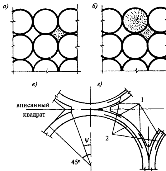
Черт. 6. К расчету звездочки
