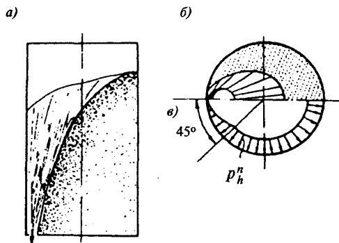
Черт. 3. Пристенный выпуск зерна
