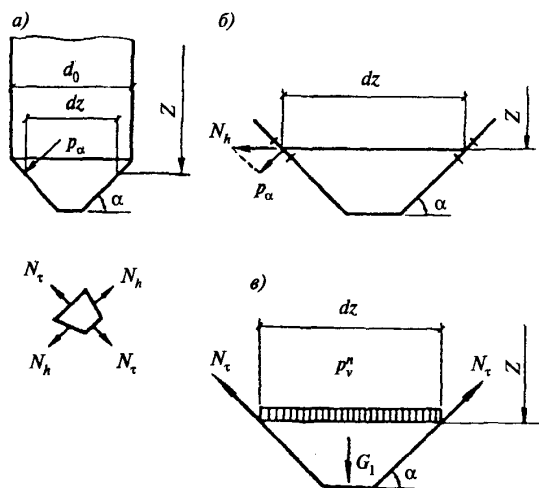
Черт. 7. Расчетные схемы конической воронки
