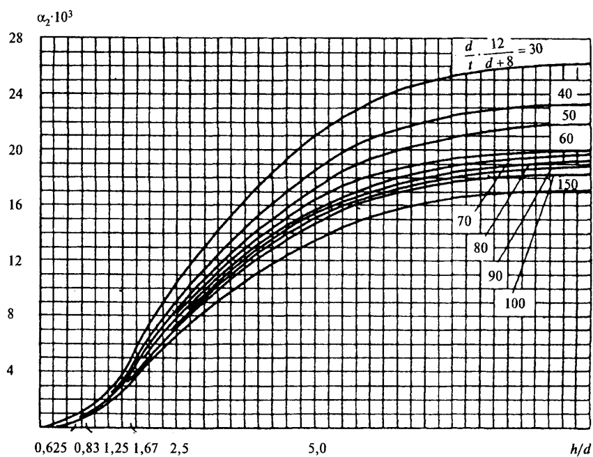
Черт. 5. Значения коэффициента \alpha_2
