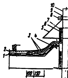
Рис 3. Пример решения пропуска трубы
