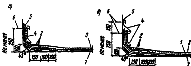
Рис 1 Примеры примыканий кровель
