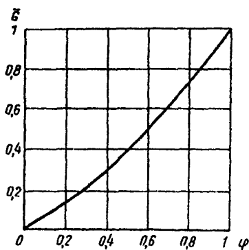
Рис. 1. График расхода теплоносителя при количественном регулировании отопительной нагрузки ( t_r'' = 80\text{ }^{\circ}\text{C} , t_o'' = 35\text{ }^{\circ}\text{C} , t_b = 18\text{ }^{\circ}\text{C} )
