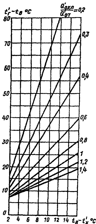
Рис. 7. Зависимость температуры теплоносителя от температуры хладоносителя и соотношения холодо- и тепловых нагрузок для радиационных систем отопления
