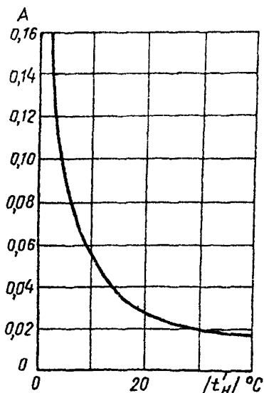
Рис. 3. Эмпирический коэффициент A для определения доли пикового подогрева
