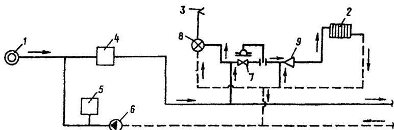
Рис. 10. Принципиальная схема бессливной системы геотермального теплоснабжения
