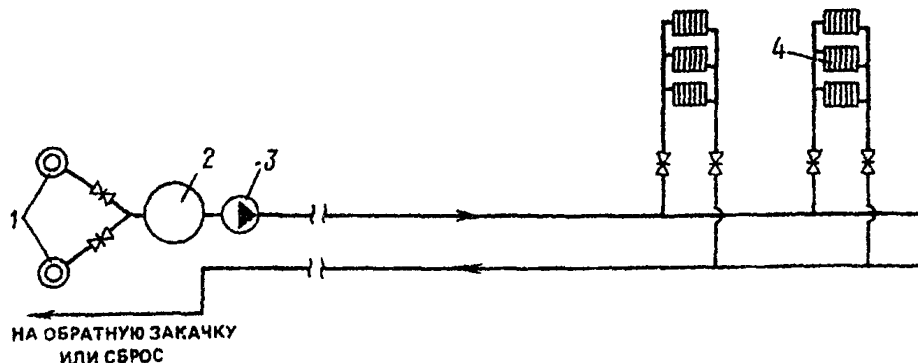
Рис. 9. Геотермальная система теплоснабжения с зависимым присоединением отопления (ГВ отсутствует) 1 — геотермальные скважины; 2 — промежуточный бак-аккумулятор геотермальной воды; 3 — сетевой насос; 4 — отопительные приборы
