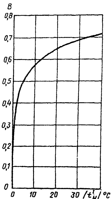
Рис. 4. Эмпирический коэффициент B для определения доли пикового подогрева
