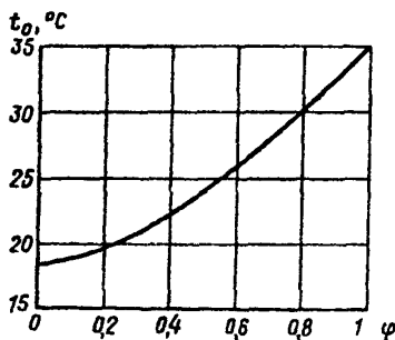
Рис. 2. График температуры обратной воды при количественном регулировании отопительной нагрузки ( t_r'' = 80\text{ }^{\circ}\text{C} , t_o'' = 35\text{ }^{\circ}\text{C} , t_b = 18\text{ }^{\circ}\text{C} )
