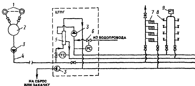
Рис. 6. Закрытая однетрубная геотермальная система теплоснабжения с зависимым присоединением отопления (распределительная сеть четырехтрубная)
