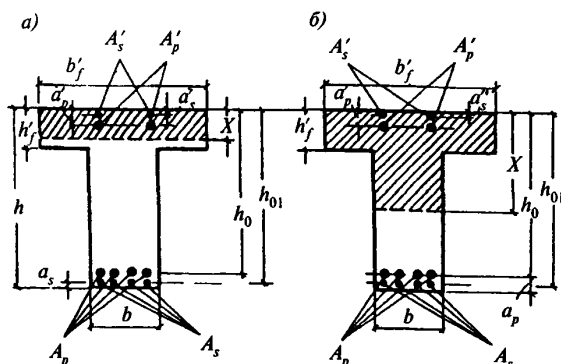
Черт. 3. Форма сжатой зоны в сечениях железобетонных элементов с плитой в сжатой зоне
