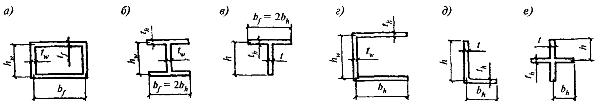
Черт. 11. Схемы расчетных сечений элементов, не подкрепленных ребрами жесткости
