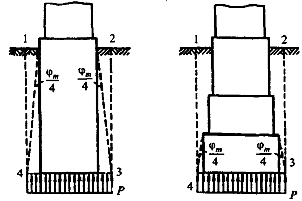
Черт. 5. Условный фундамент из опускающего колодца а — без уступов; б — с уступами
