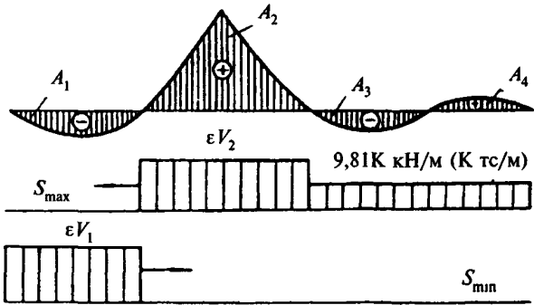
Черт. 5. Схема загрузки участков линии влияния для определения максимальных и минимальных усилий (напряжений) при расчете на выносливость
