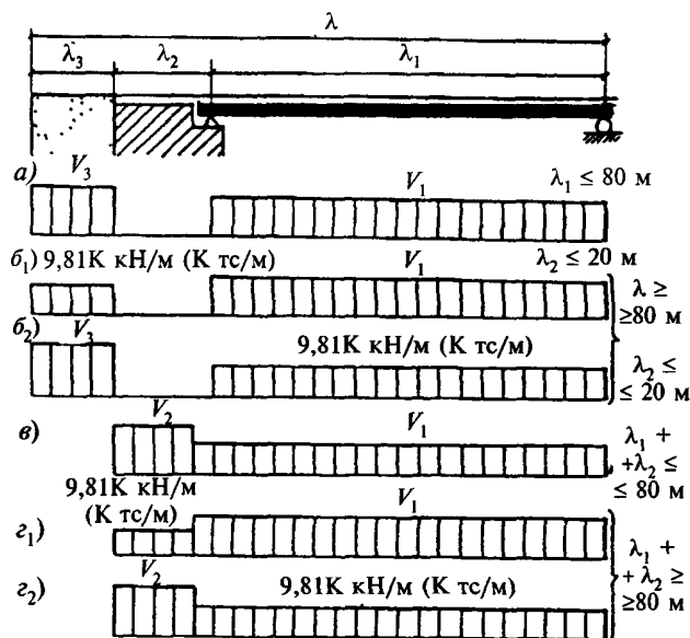
Черт. 4. Схема загрузки пролета одновременно с призмой обрушения или пролета с устоем при расчете массивных устоев мостов с разрезными балочными пролетными строениями
