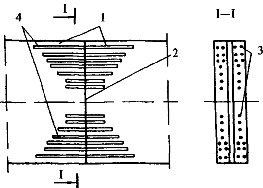
Черт. 18. Клеештыревой стык
