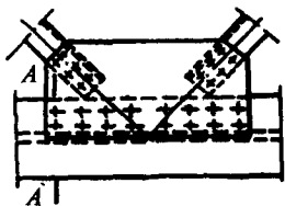
Черт. 3. Расположение проверяемого на выносливость расчетного сечения А—А по основному металлу в сечении брутто по первому ряду высокопрочных болтов в прикреплении фасонки к жесткому в данном узле поясам сплошных балок и элементам решетчатых ферм
