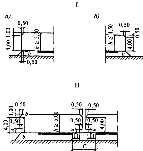
Условные обозначения: а — П принимается по п. 2*; б — бровка земляного полотна, б — определяется конструкцией ограждающих устройств Черт. 3. Схемы габаритов приближения конструкций под путепроводами I — при отсутствии ограждений на пересекаемых дорогах, II — при наличии опор на разделительной полосе и ограждений на дороге; а — категорий I—III, III-п и IV-п; б — категорий IV и V
