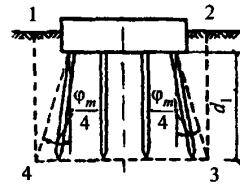
Черт. 1. Условный свайный фундамент с ростверком, заглубленным в грунт при угле наклона свай менее \varphi_m/4
