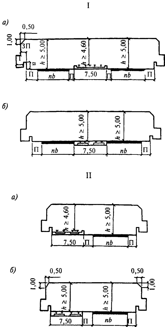
Черт. 2. Схемы габаритов приближения конструкций на городских мостах с трамвайным движением I — трамвайные пути расположены на оси моста; II — трамвайные пути смещены относительно оси моста, а — на обособленном полотне; б — на общем полотне
