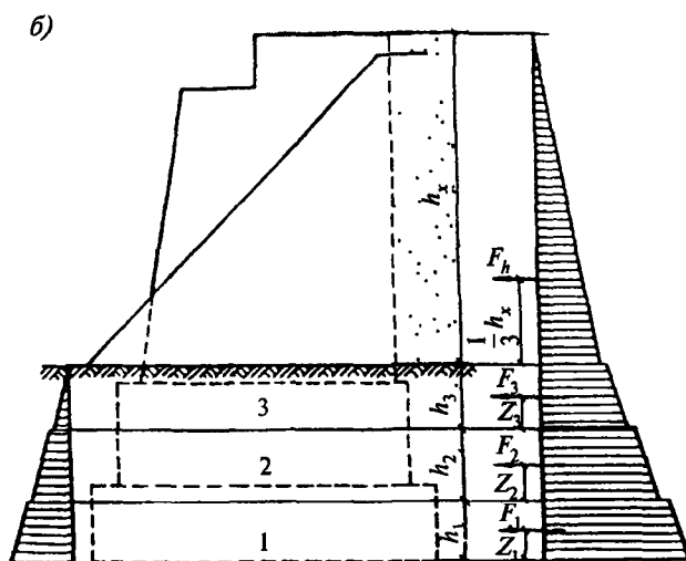
Схема эпюр давления грунта на опоры моста для определения равнодействующей нормативного горизонтального (бокового) давления на опоры
