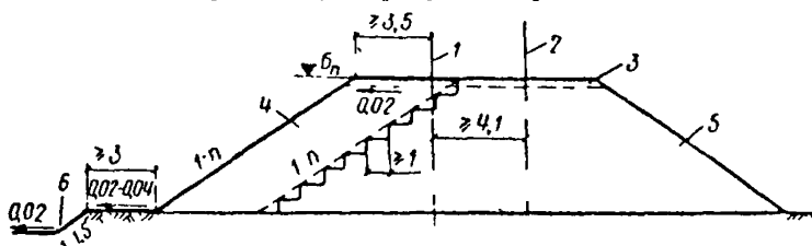
Рис. 37. Поперечный профиль насыпи, ушляемой под второй путь 1 — ось второго пути; 2 — ось существующего пути; 3 — дренарующий грунт; 4 — проектируемая присыпка; 5 — существующая насыпь; 6 — резерв или канава
