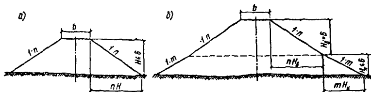
Рис. 3. Поперечные профили насыпей высот:
