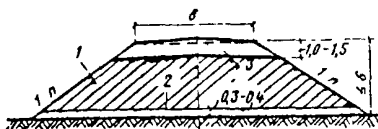
Рис. 13. Поперечный профиль насыпей из глинистых переувлажненных грунтов для автомобильных дорог
