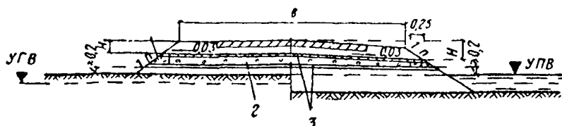
Рис. 11. Поперечные профили автодорожных насыпей с капилляропрерывающей прослойкой
