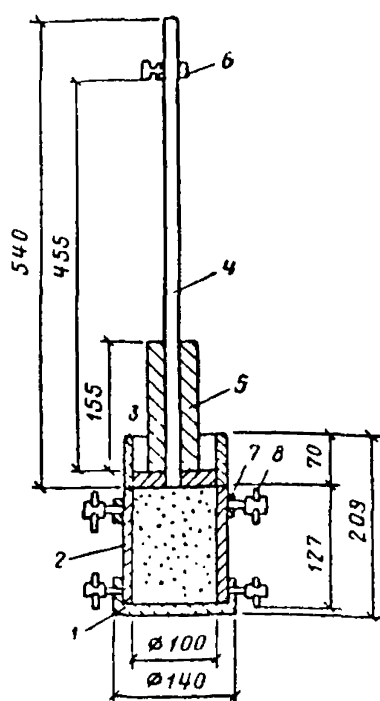
Рис. 41. Схема прибора Союздорнии для стандартного уплотнения грунтов
