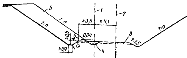
Рис. 38. Поперечный профиль выемки, уширяемой под второй путь
