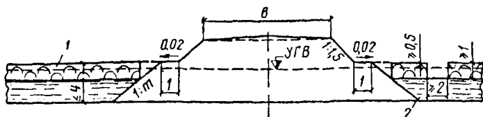
Рис. 30. Поперечный профиль автодорожных насыпей на болотах III типа
