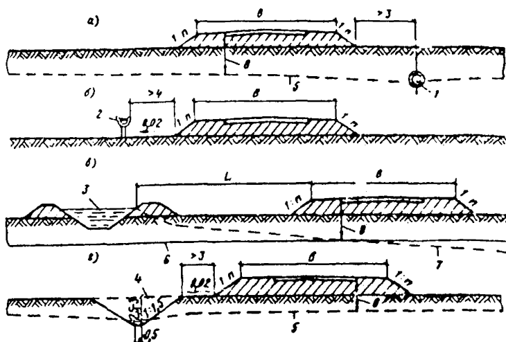
Рис. 35. Поперечные профили насыпей вблизи ирригационных сооружений
