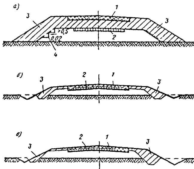
Рис. 39. Поперечные профили земляного полотна реконструируемых автомобильных дорог
