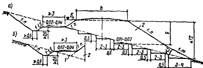
Рис. 4. Поперечный профиль насыпей из недренирующих грунтов для железных дорог на косогорах крутизной от 1:5 до 1:3
