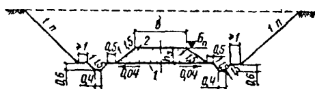
Рис. 19. Поперечный про- филь выемок для желе- зных дорог в переувлаж- ненных глинистых грун- тах
