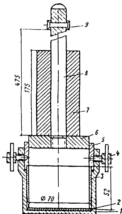
Рис. 42. Схема прибора ЦНИИС для стандартного уплотнения грунтов
