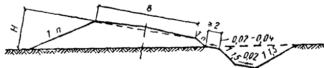
Рис. 8. Поперечный профиль насыпей из грунта бокового резерва для автомобильных дорог на косогорах крутизной от 1:10 до 1:5
