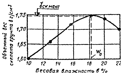
Рис. 43. Кривая стандартного уплотнения
