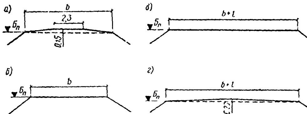
Рис. 2 Поперечное очертание верха земляного полотна.
