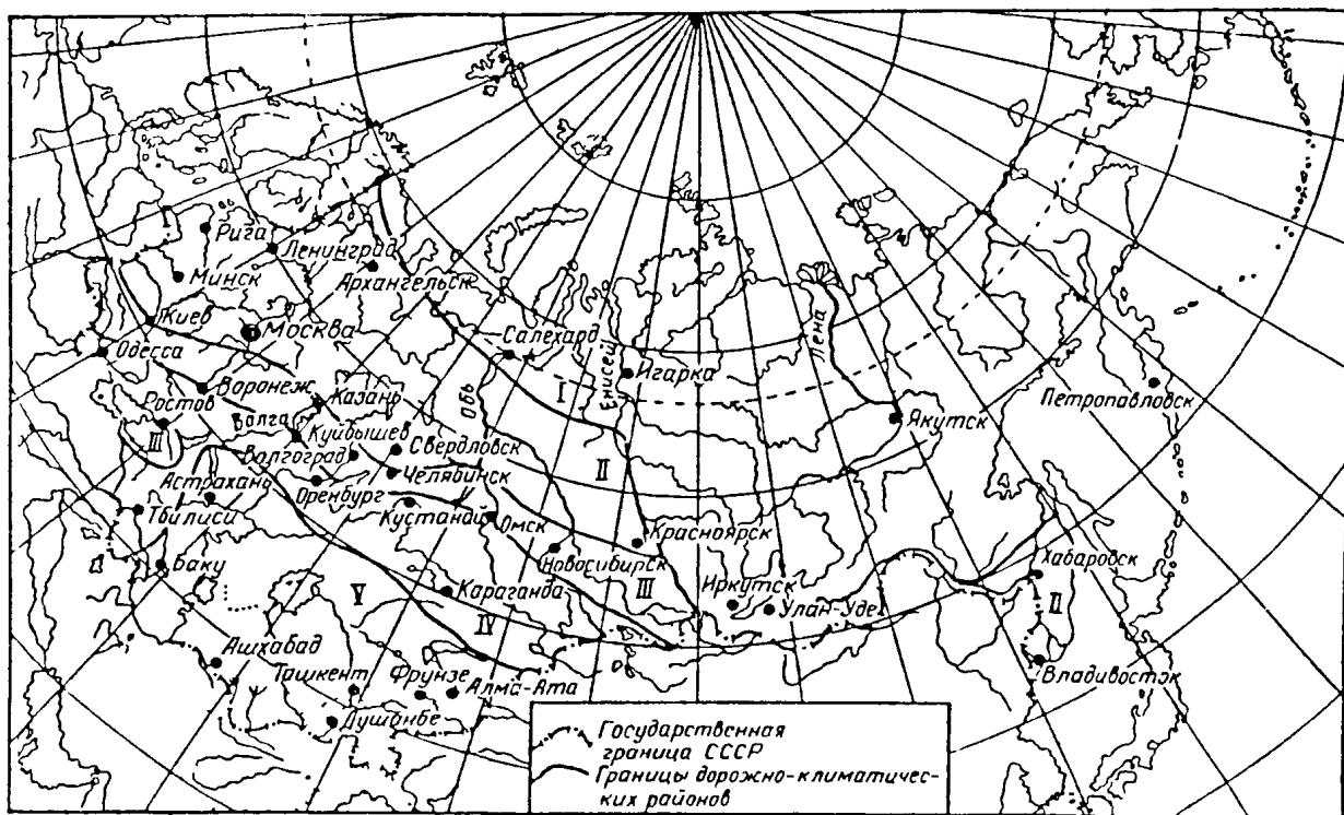
Рис. 1 Схема деления территории СССР на дорожно-климатические зоны
