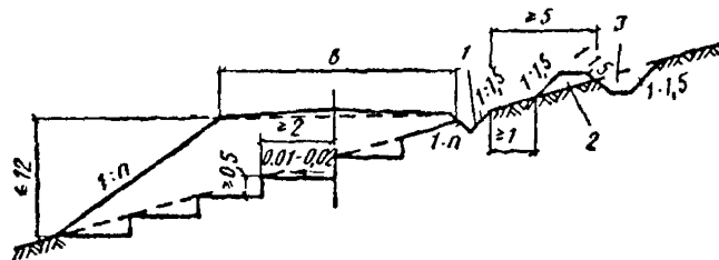
Рис. 9. Поперечный профиль насыпей для автомобильных дорог на косогорах крутизной от 1:5 до 1:3 1 — кювет глубиной не менее 0,3 м; 2 — банкет, 3 — нагорная канава
