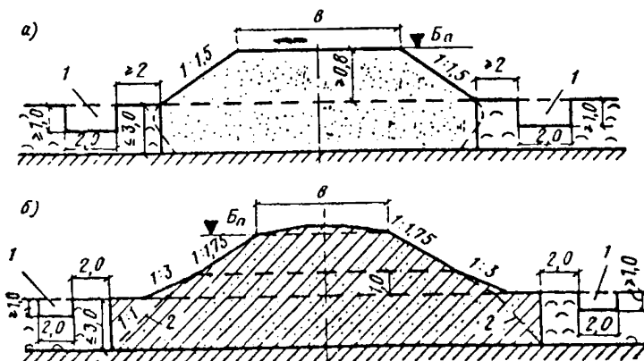
Рис. 27. Поперечные профили железнодорожных насыпей на болотах II типа
