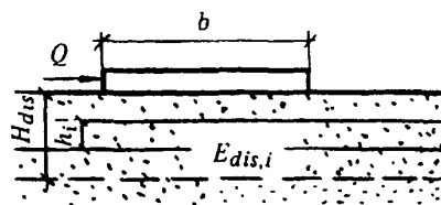
Черт. 1. Схемы к определению горизонтальных смещений сооружений
