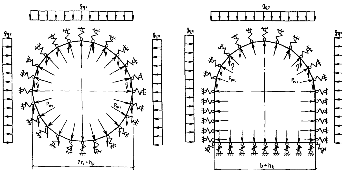
Черт. 1. Расчетные схемы обделок туннелей
