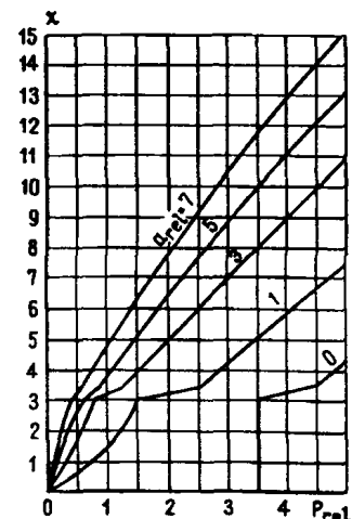
Черт. 3. График зависимости коэффициента \chi от p_{rel} при a_{rel} = \text{const}
