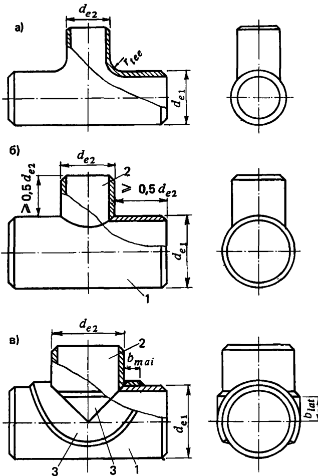
Черт. 1. Тройники
